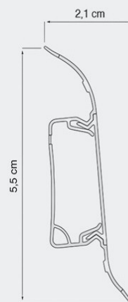
- Profil lišty IZZI – technický řez
