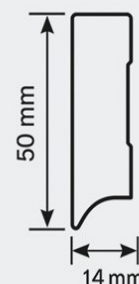
– Profil lišty RIGID RS 50 – technický řez
