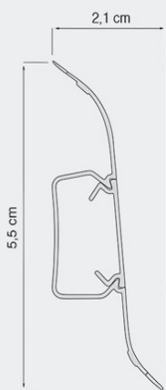
- Profil lišty SMART FLEX – technický řez
